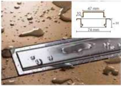
Schlüter®-KERDI-LINE-A
